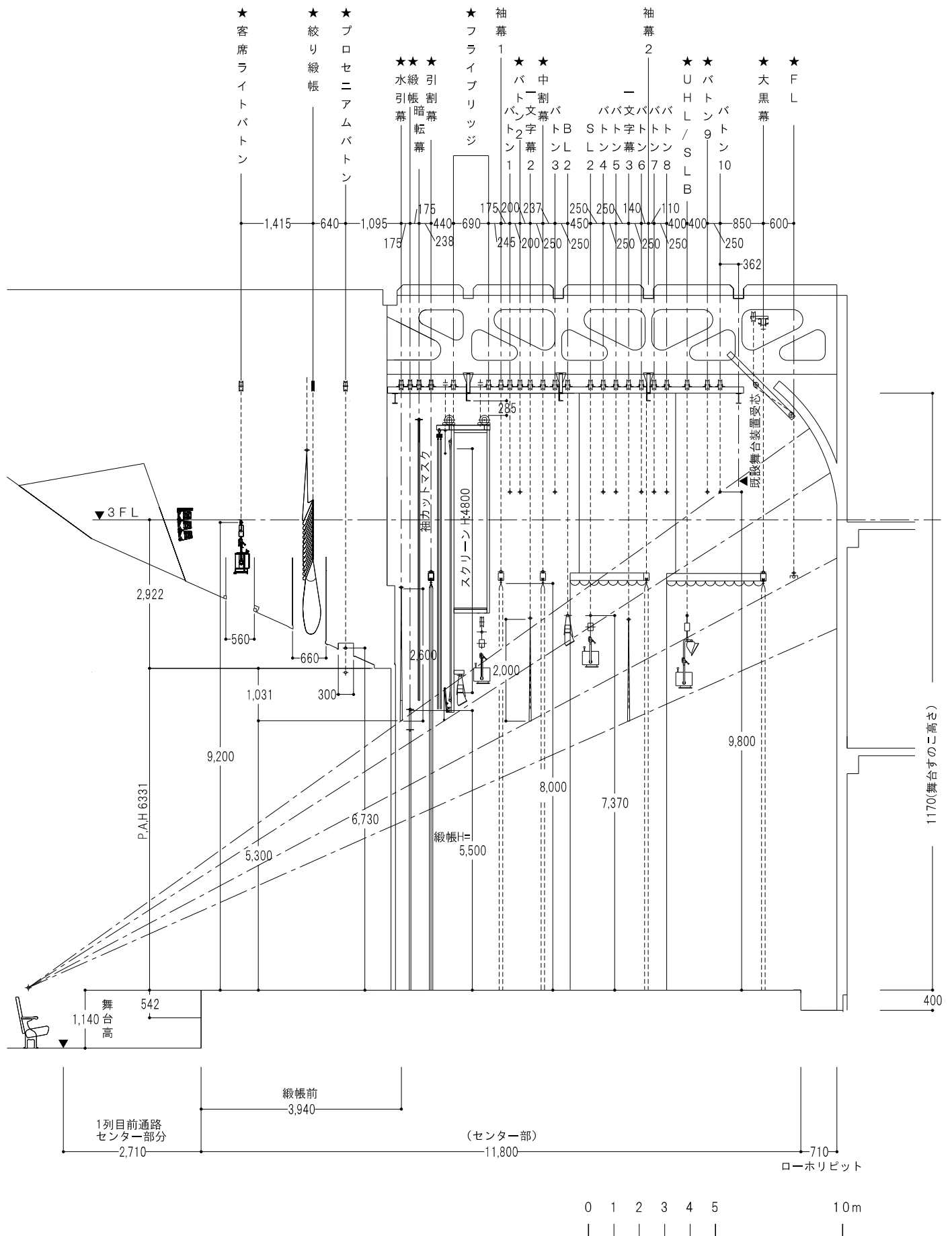
名古屋市公会堂 大ホール舞台断面図
